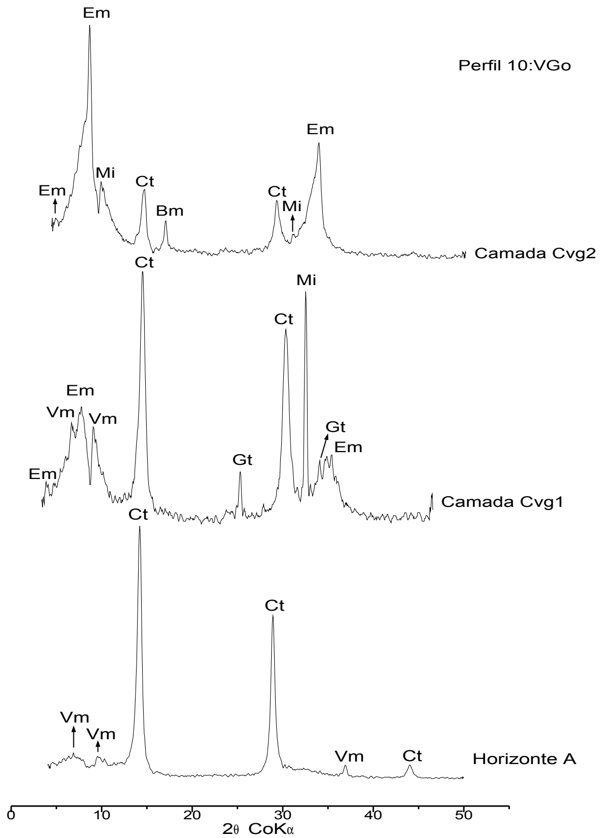
Figura 24 - Difratoogramas de raios-X da fração argila do VGo, perfil 10. Em-esmectita; Ct-caulinita; Vm-vermiculita; Gt-goethita; Bm-boemita; Mi-mica.
