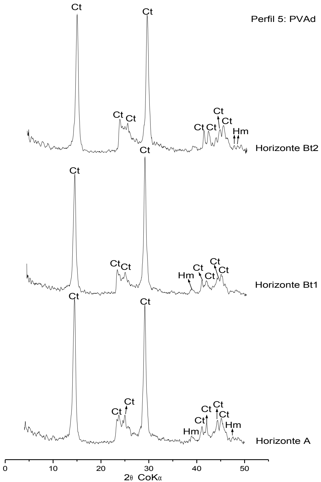
Figura 15 - Difratoigramas de raios-X da fração argila do PVAd, perfil 5, horizontes A, Bt1 e Bt2. Ct-caillinita; Hm-hematita.
