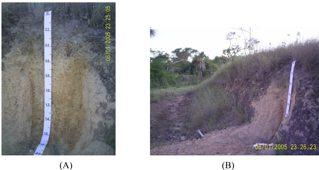
Figura 16 - Perfil de Plintossolo Pétrico, mostrando profundidade, presença de petroplintitas (A) e trincheira inserida na paisagem em relevo ondulado (B).
