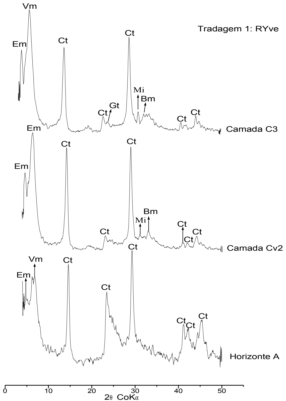
Figura 26 - Difratogramas de raios-X da fração argila do RYve, tradagem 2 próxima ao perfil 12. Em-esmectita; Ct-caulinita; Vm-vermiculita; Mi-mica; Bm-boemita; Gt-goethita.
