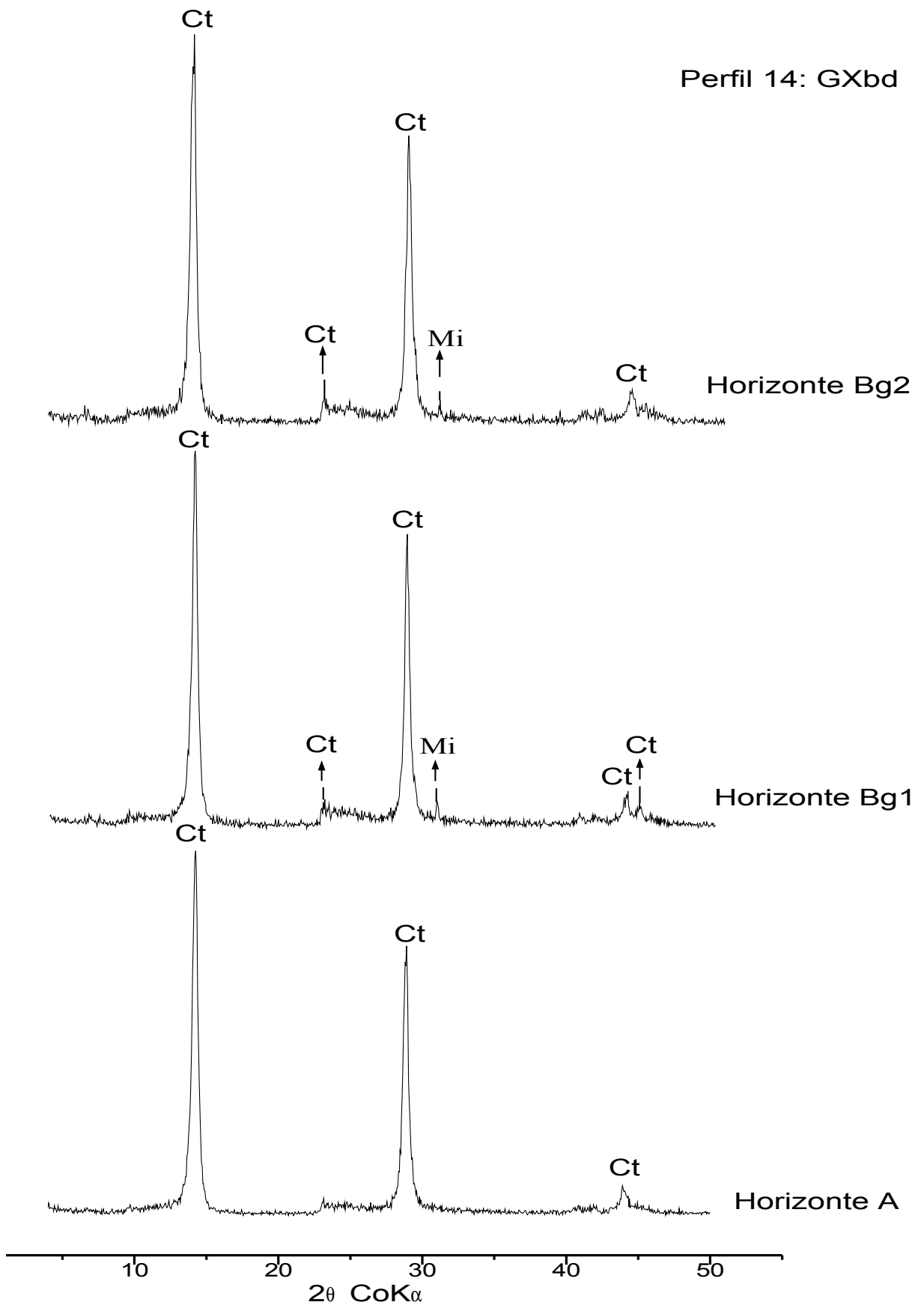
Figura 21 - Difratogramas de raios-X da fração argila do GXbd, perfil 14, horizontes A, Bg1 e Bg2. Ct-caulinita; Mi-mica.
