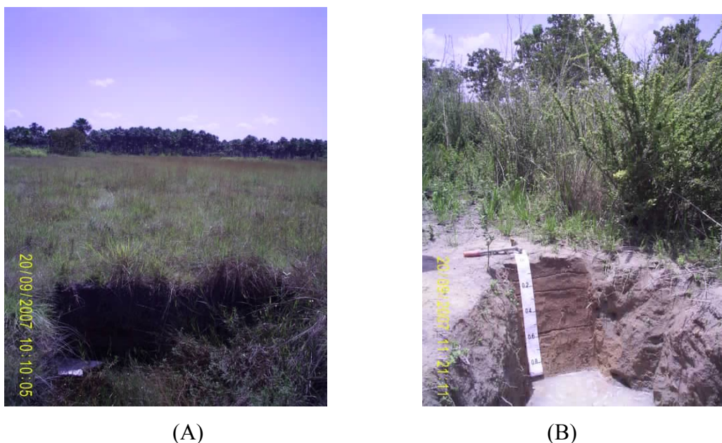
(A) (B) Figura 18 - Gleissolo Háptico típico (perfil 13 - A) e Gleissolo Háptico Plíntico (perfil 14 - B), inseridos na paisagem de vegetação do tipo formação pioneira em relevo abaciado.
