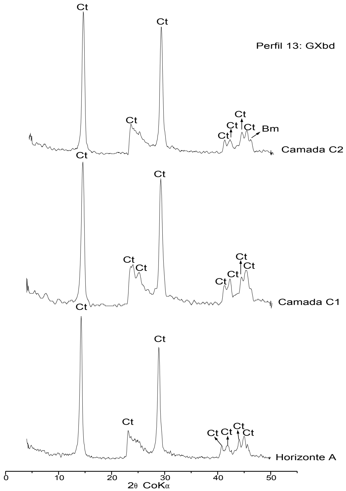
Figura 20 - Difratoformas de raios-X da fração argila do GXbd, perfil 13, horizontes A, Bg1 e Bg2. Ct-caulinita; Bm-boemita.
