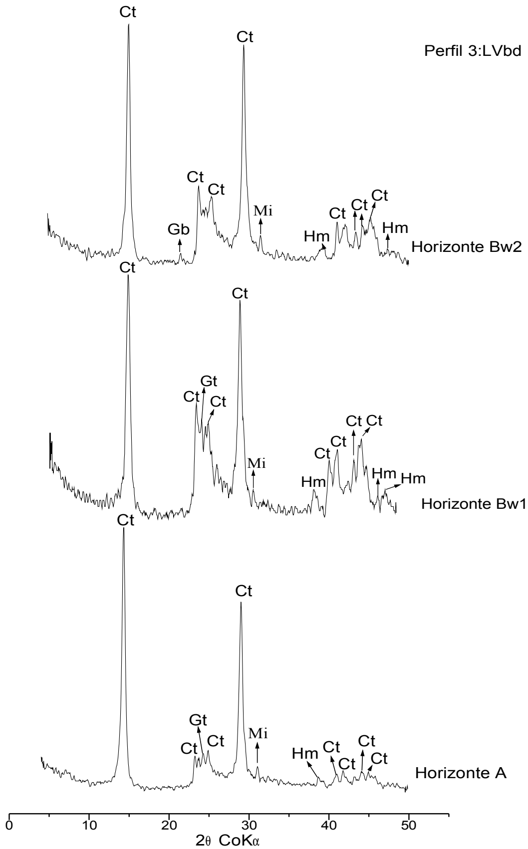
Figura 13 - Difratoformas de raios-X da fração argila do LVd, perfil 3. Ct-caulinita; Hm-hematita; Mi-mica; Gt-goethita; Gb-gibsite.
