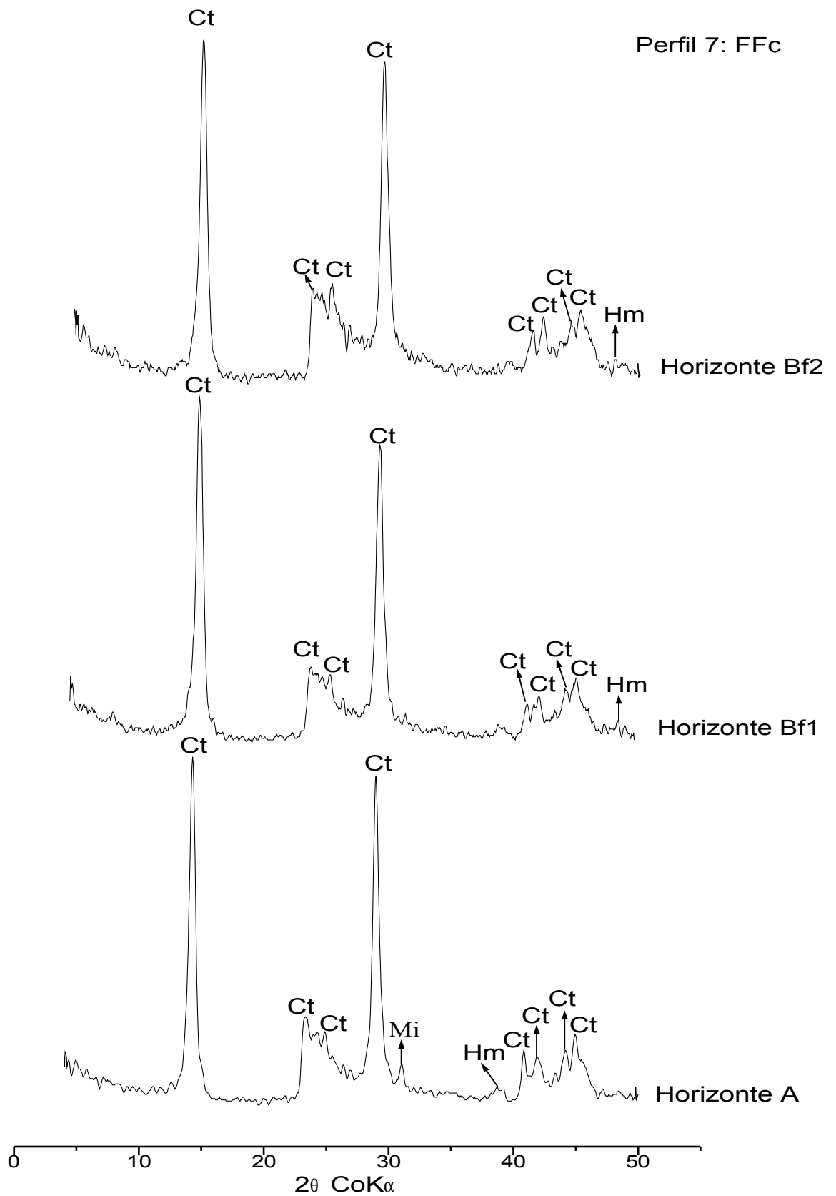
Figura 17 - Difratoformas de raios-X da fração argila do FFc, perfil 7, horizontes A,
