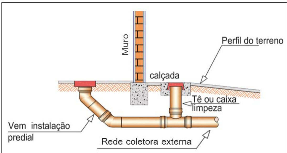
Figura 12 – Tubulações e dispositivos que fazem parte do sistema de esgoto.
