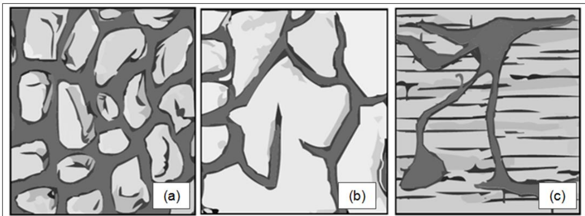
Figura 3 – (a) Aquíferos porosos, (b) Aquíferos fissural ou fraturado, (c) Aquíferos cársticos.
