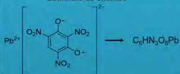
Estifinato de chumbo
