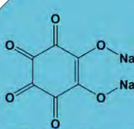
Rodizonato de sódio
